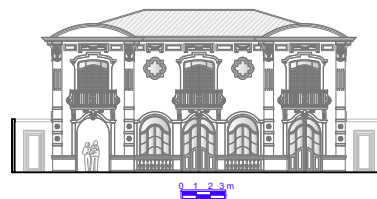
Elevação 03
