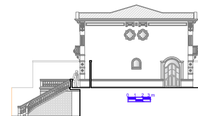
Elevação 04
