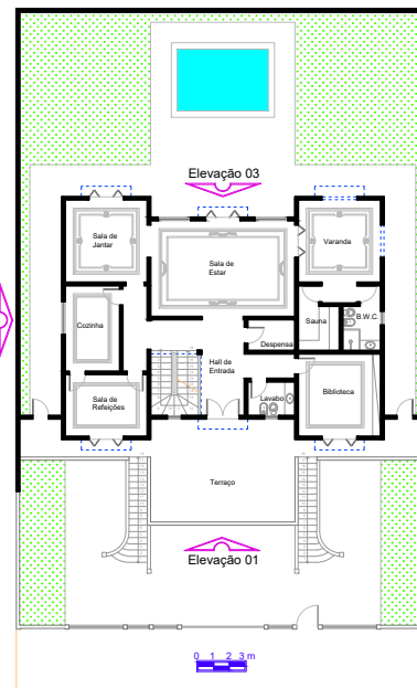
Térreo A = 165,34 m 2
