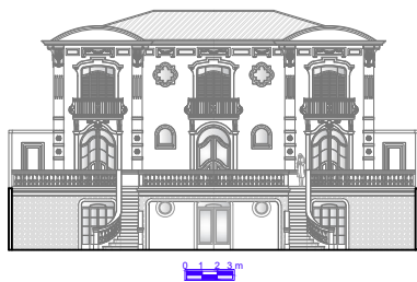
Elevação 01
